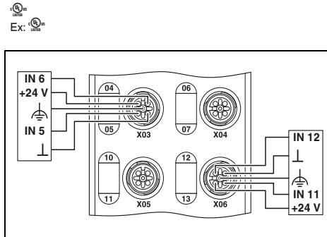
16 digital inputs
